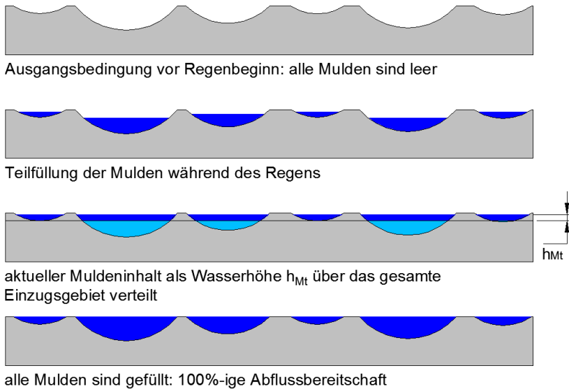
Abbildung 26: Prinzip der Muldenverluste
