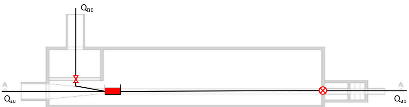
Abbildung 84: Fangbecken im Hauptschluss - Hydrodynamische Modellierung (hydraulisch)
