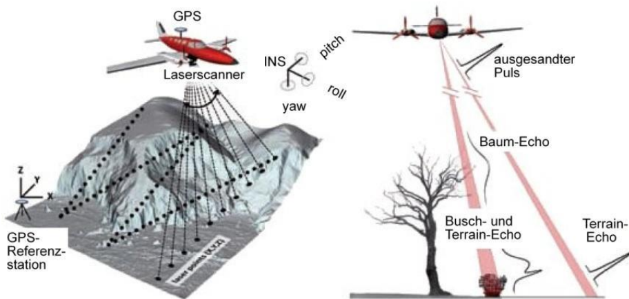
Abbildung 3: Prinzip des Airborne Laserscanning (de LANGE, 2013)
