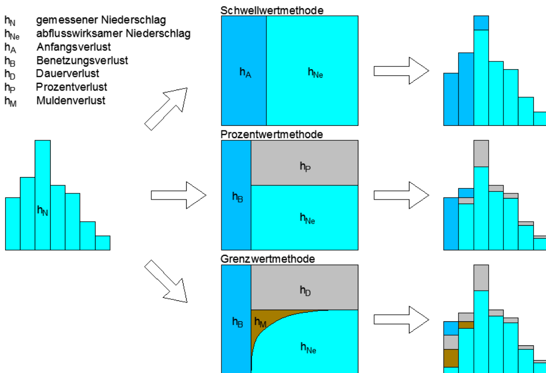
Abbildung 22: Abflussbildungsansätze
