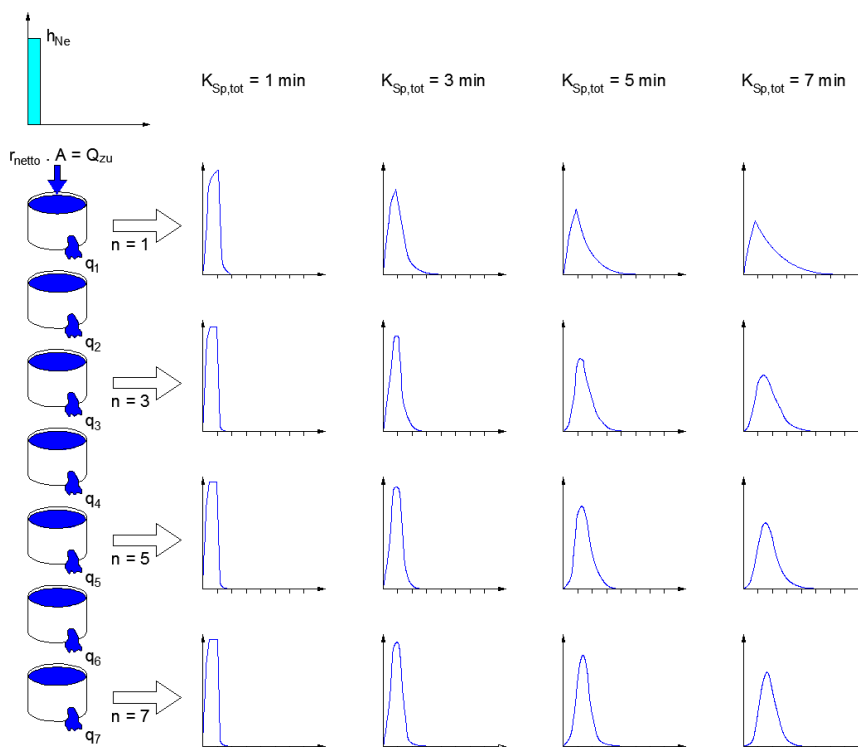
Abbildung 37: Schematische Darstellung der Linearspeicherkaskade
