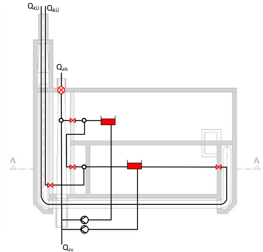
Abbildung 91: Verbundbecken im Nebenschluss - Hydrodynamische Modellierung (hydraulisch und stofflich)
